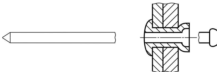
Рисунок 6 — Сердечник с отрывающейся головкой
