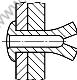
Рисунок 15 — Разделяющийся конец
