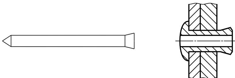
Рисунок 4 — Сердечник, протягиваемый насквозь
