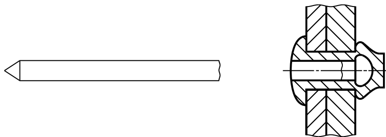
Рисунок 13 — Закрытый конец
