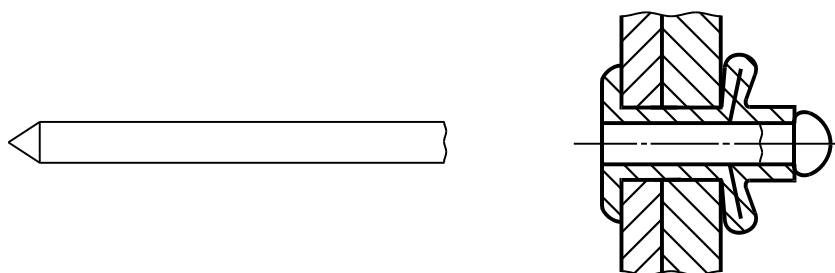
Рисунок 16 — Разрезной стержень
