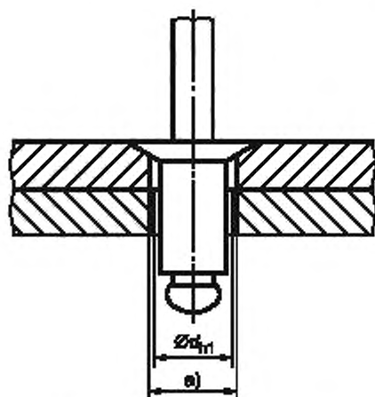
Рисунок 2 — Увеличенное отверстие с зазором
